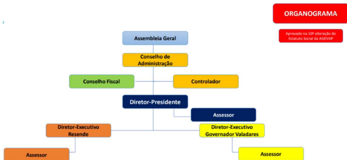
Figura 1 – Estrutura AGEVAP
