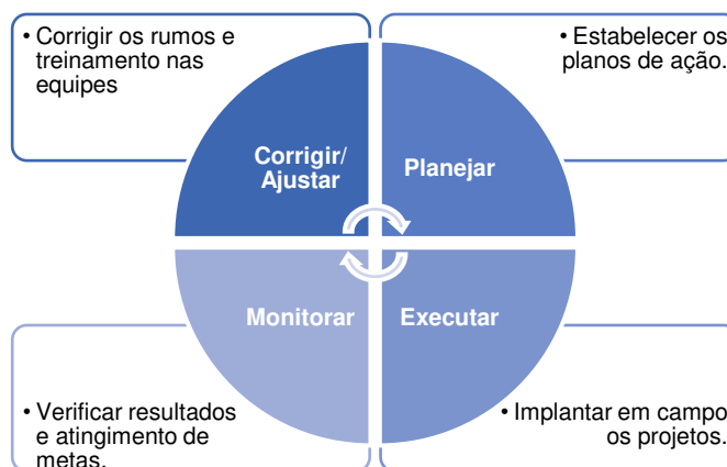
Figura 7 – Ciclo PDCA
