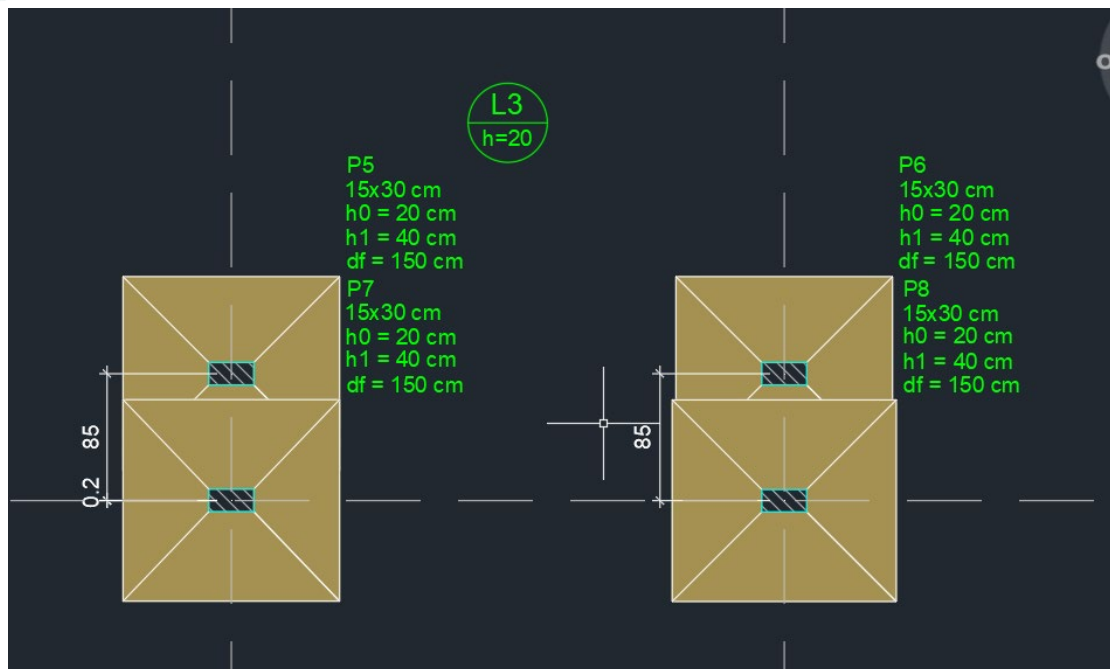
FIGURA 2 – Detalhe das sapastas apresentadas no projeto estrutural.
