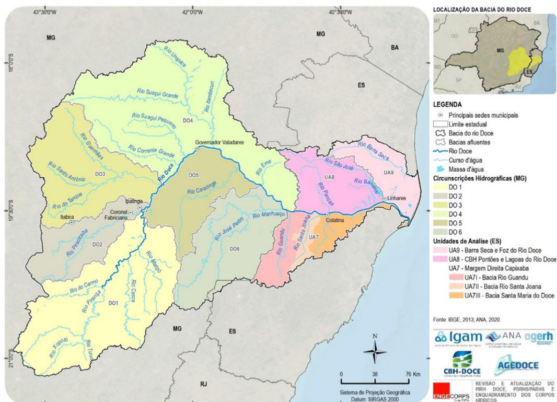
Divisões hidrográficas da bacia do rio Doce.
